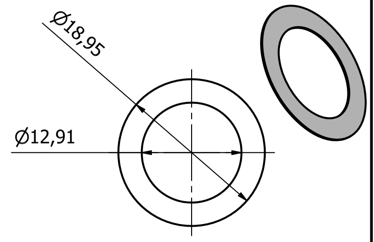
Schims T= 0,2 0,15, 0,1 & 0,05 Mässingsplåt svarvas ur plattor 21x21 i vidstående verktyg, centreras mellan hål.
