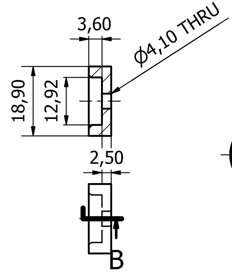
Låsbricka utvändig svarvning
