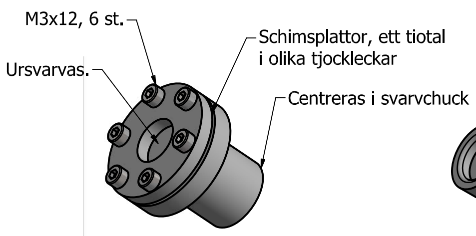
Svarvning av schims invändigt
