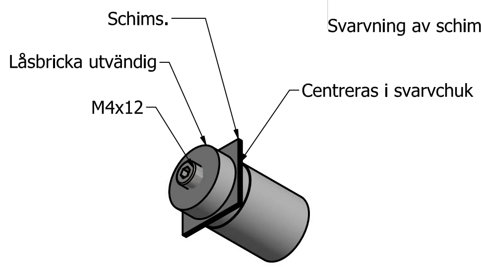
Svarvning av schims utvändigt
