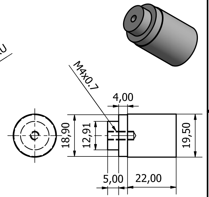
Schims T= 0,2 0,15, 0,1 & 0,05 Mässingsplåt svarvas ur plattor 21x21 i vidstående verktyg, centreras mellan hål.
